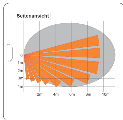
Diagramm der Erfassung auf maximaler Installationshöhe (nicht zertifiziert)
