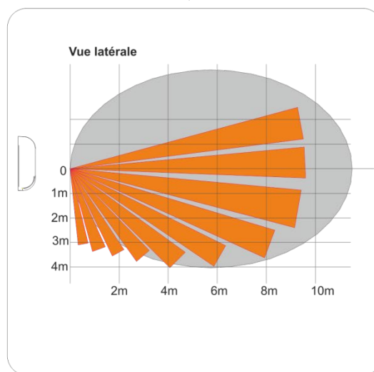
Diagramme de détection à la hauteur maximale d'installation (non certifié)
