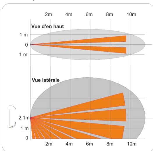
Diagramme certifié de détection
