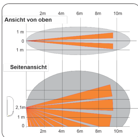
Diagramm der zertifizierten Erfassung
